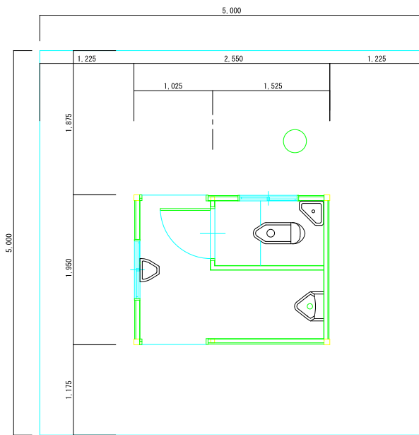
建物平面図 1/50
