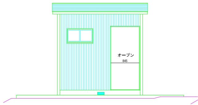
C立面図 1/50
