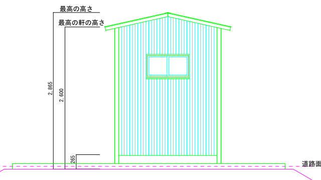
D立面図 1/50
