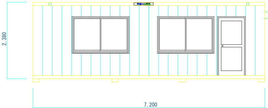
立面図
